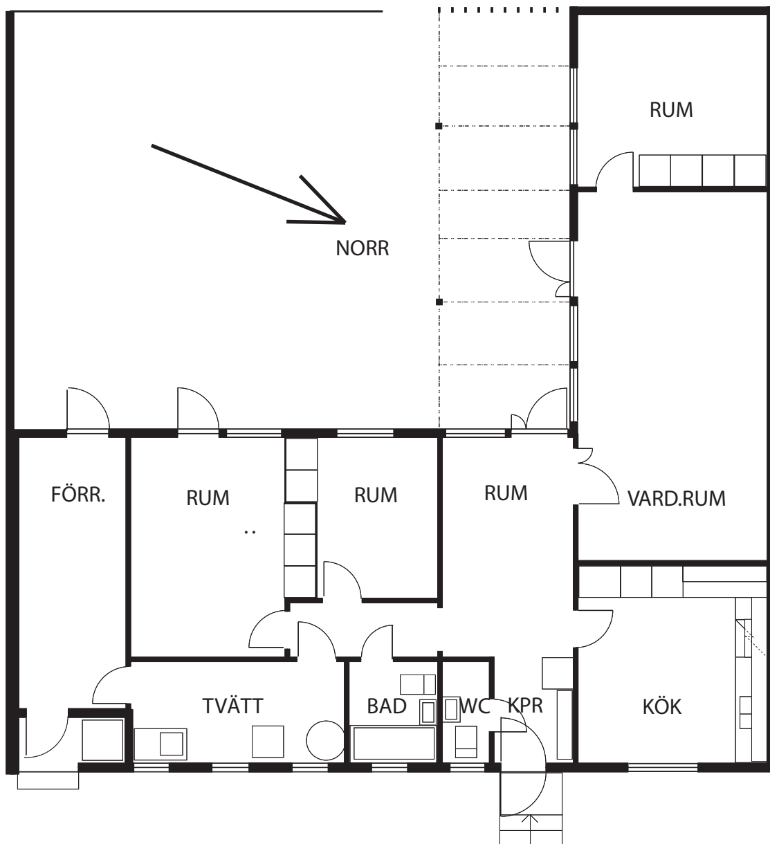
HUSTYP C Skala c 1:100
